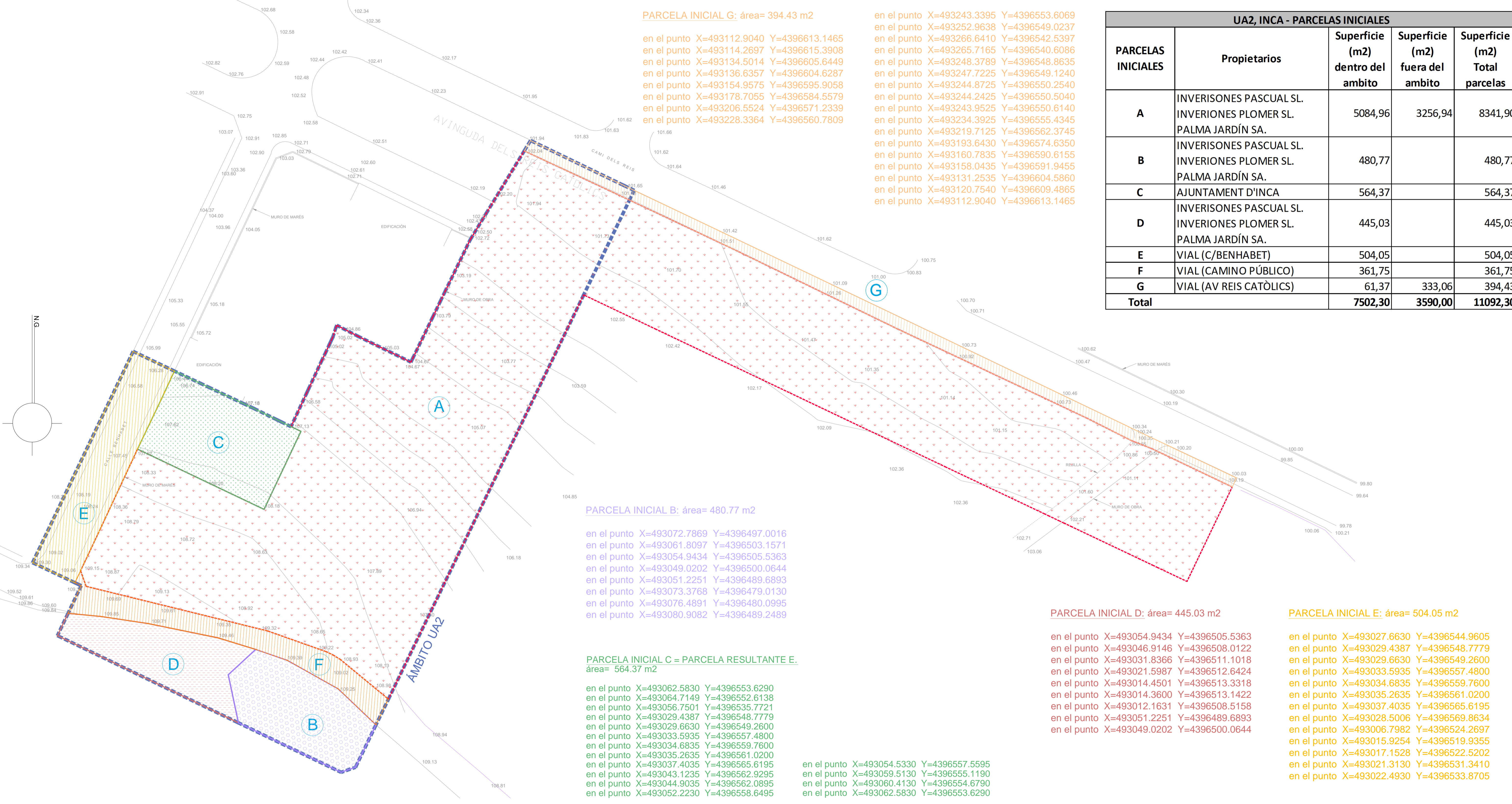
PARCELA INICIAL F: área= 361.75 m2
