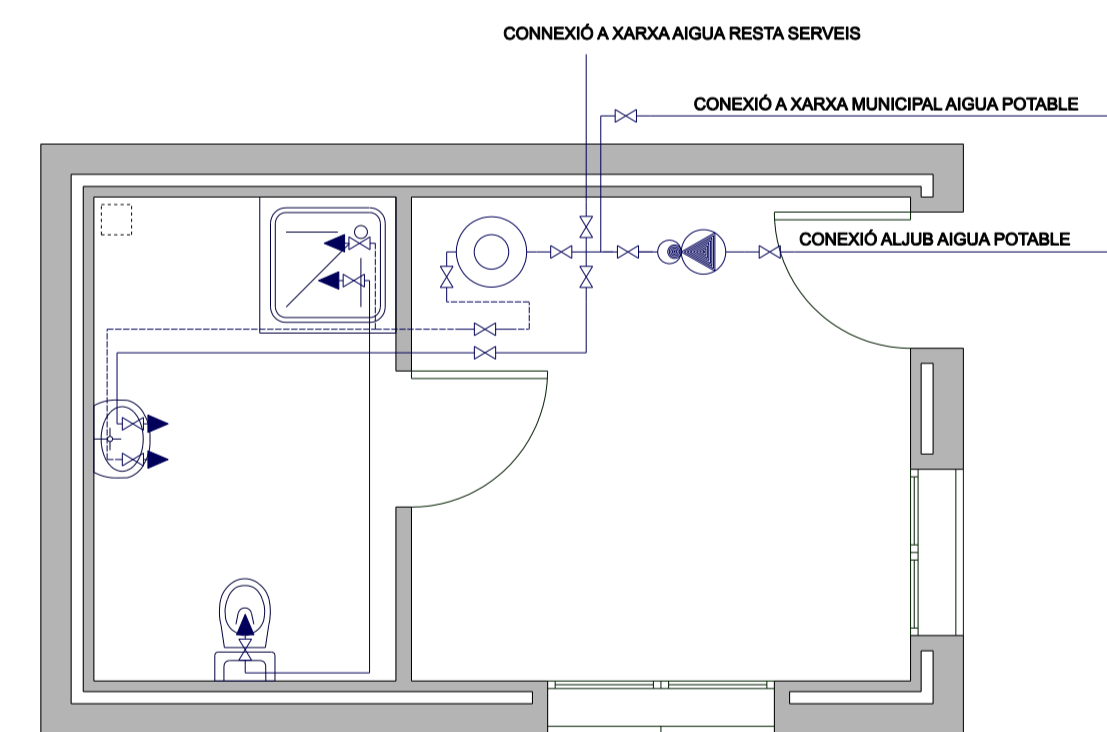
OFICINA DE RECEPCIÓ I BANY PLANTA INSTAL·LACIONS FONTANERIA
