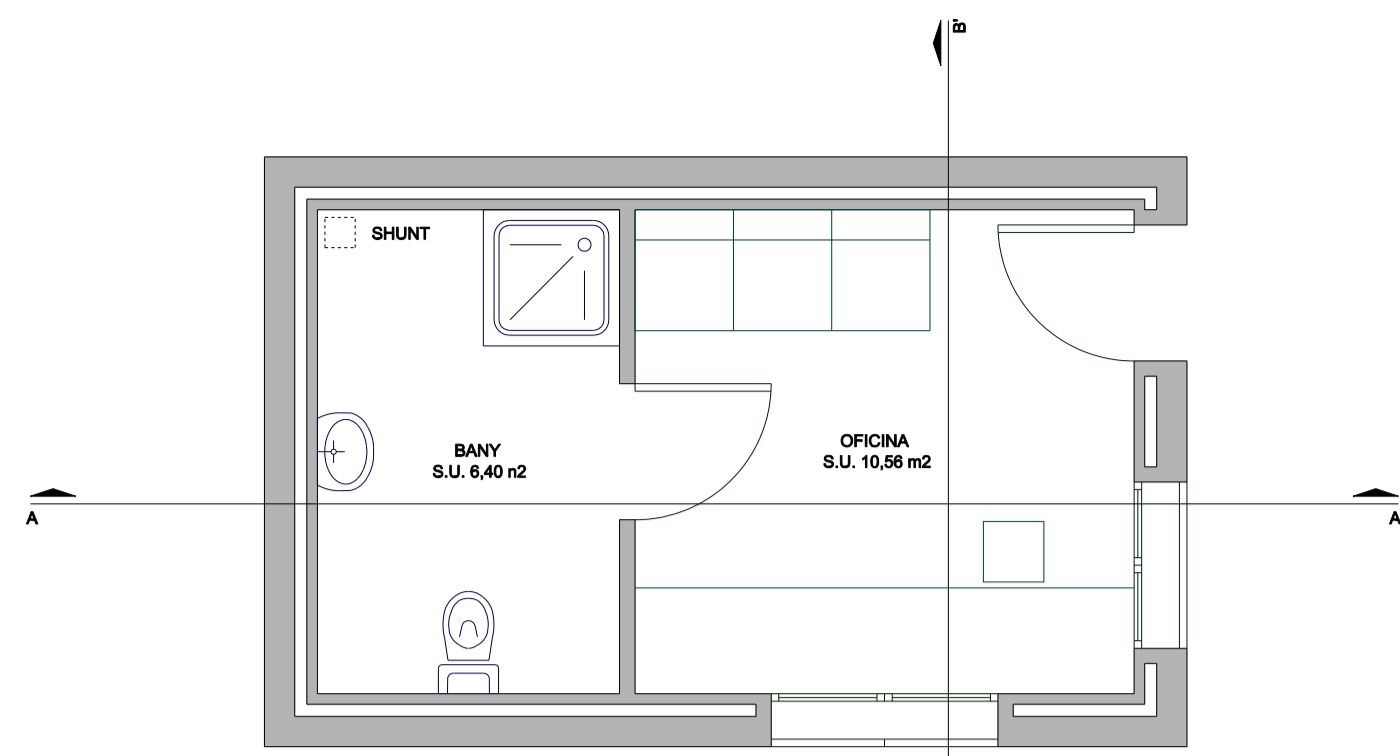
OFICINA DE RECEPCIÓ I BANY PLANTA DISTRIBUTIVA
