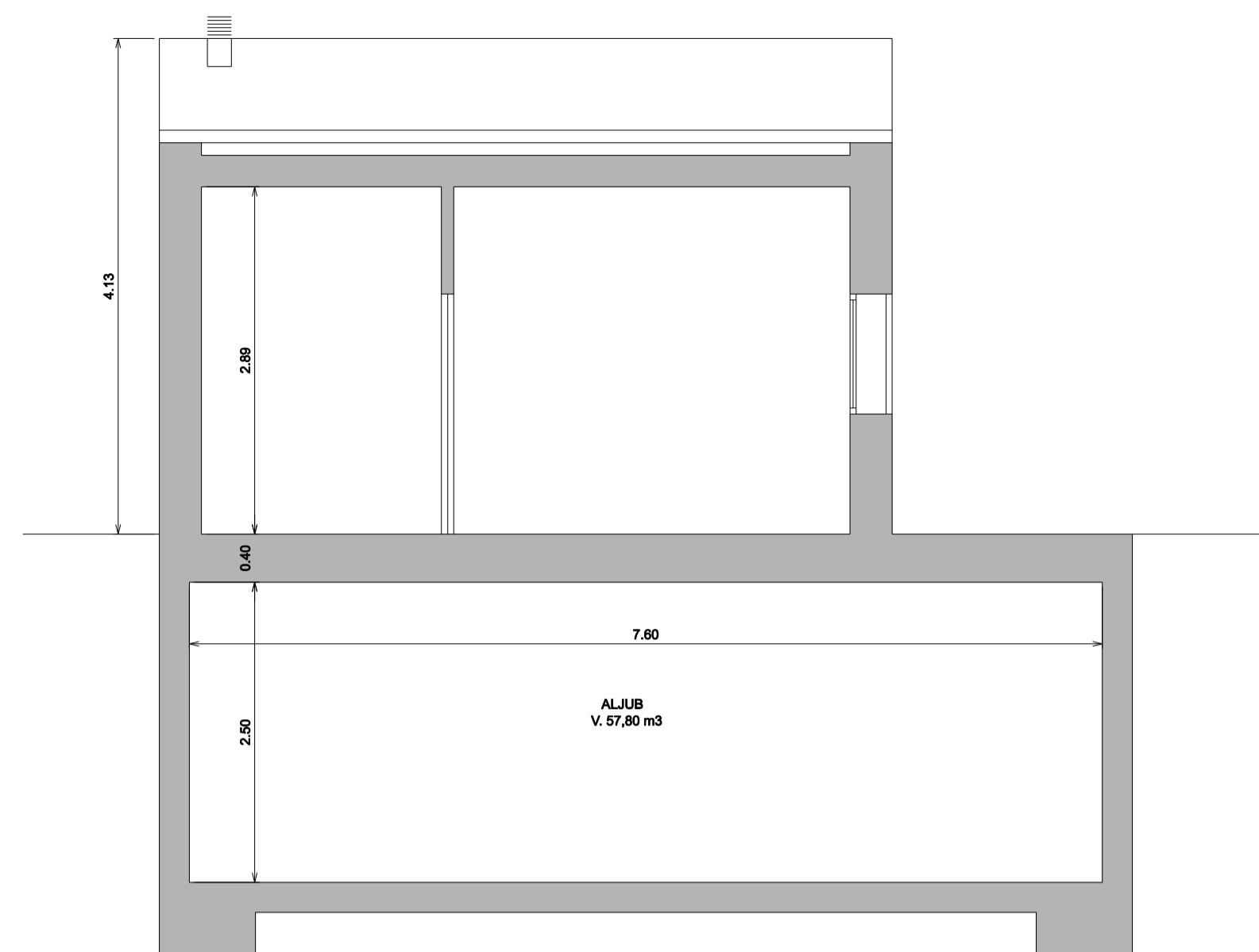
SECCIÓ A-A'
