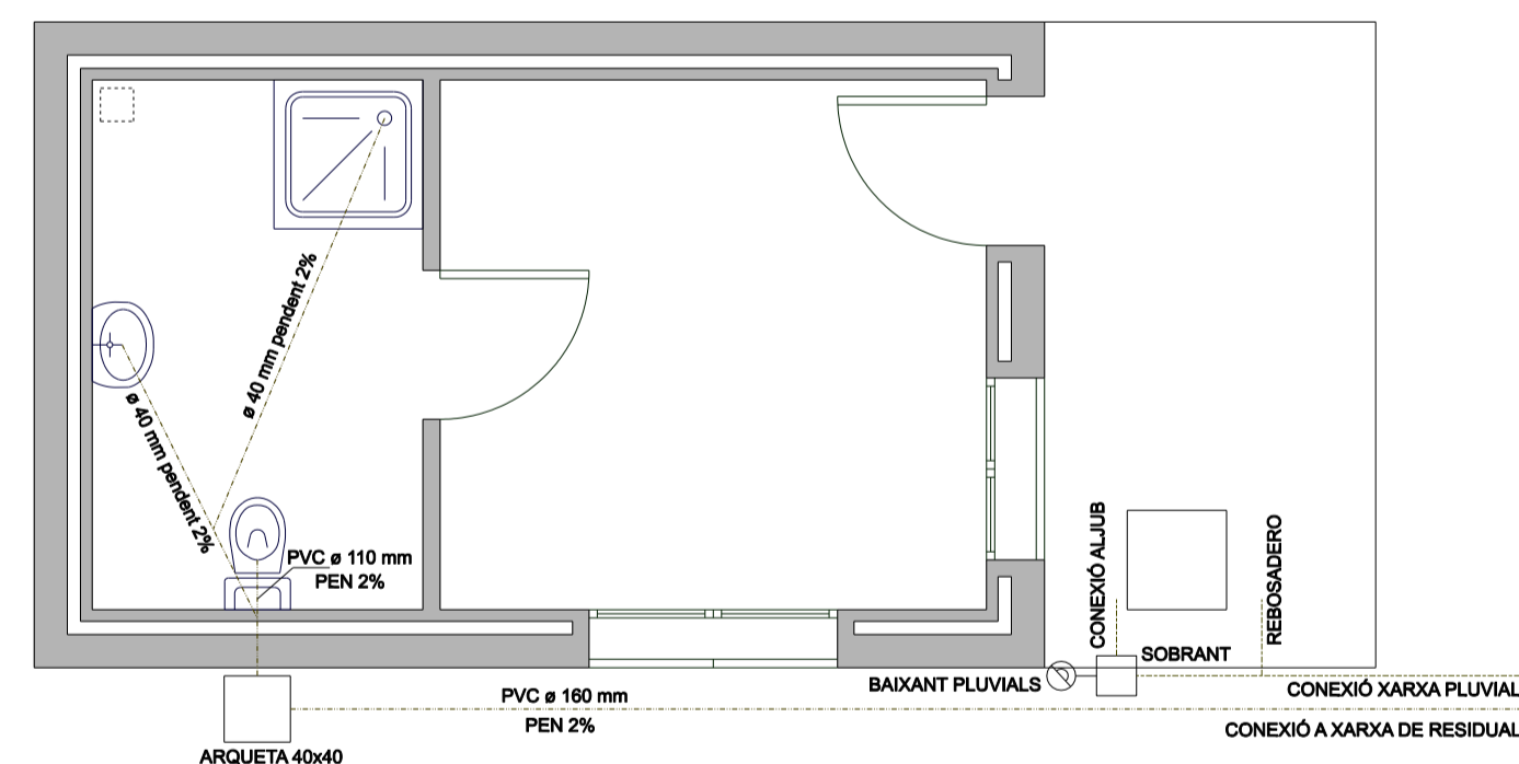
OFICINA DE RECEPCIÓ I BANY PLANTA INSTAL·LACIONS SANEJAMENT
