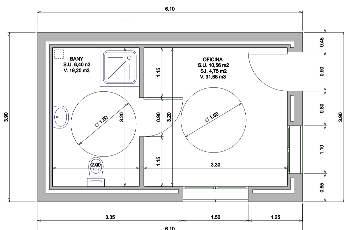
OFICINA DE RECEPCIÓ I BANY PLANTA COTES I SUPERFÍCIES SUPERFÍCIE CONSTRUÏDA TANCADA TOTAL 23,79 m 2
