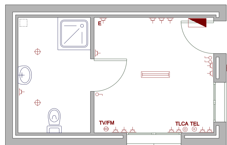
OFICINA DE RECEPCIÓ I BANY PLANTA INSTAL·LACIONS ELÈCTRIQUES
