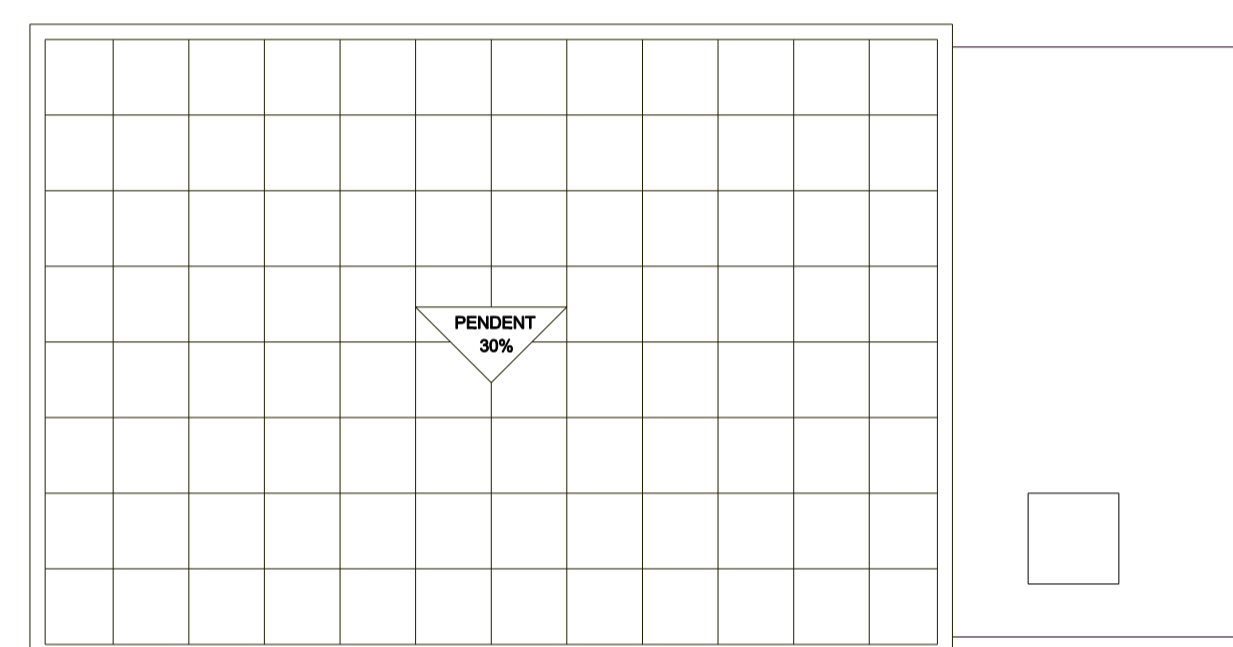
PLANTA COBERTA
