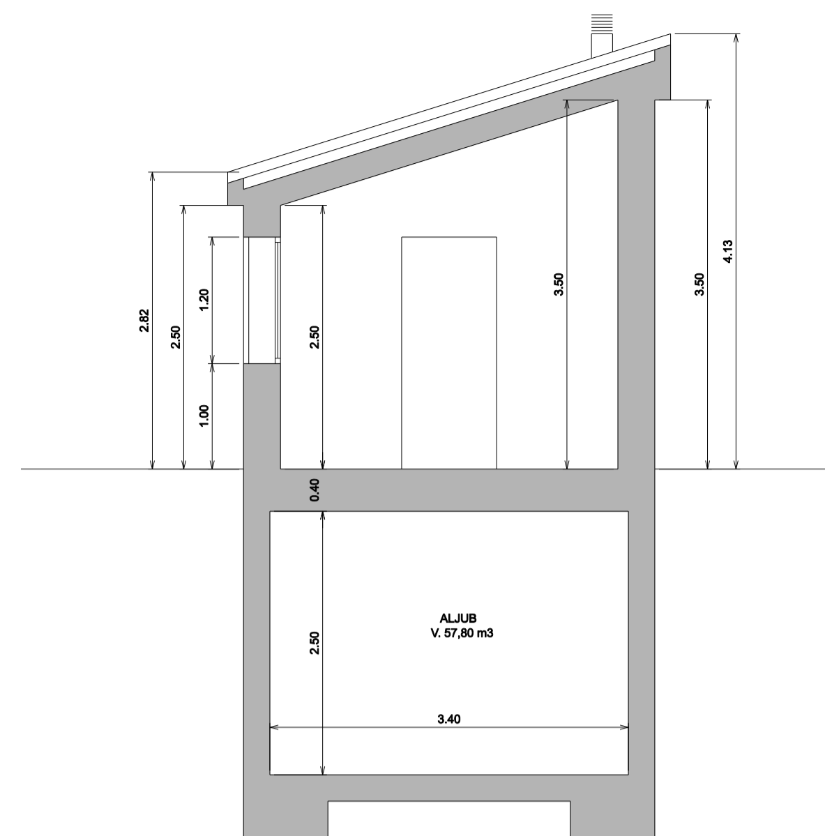
SECCIÓ B-B'
